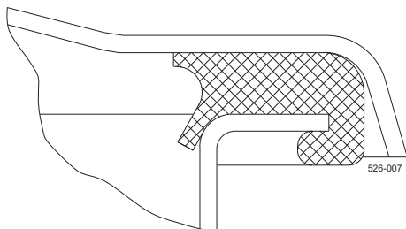
图 2. 双唇密封件
